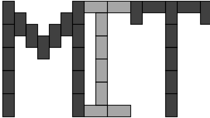
Figure 16.5: MIT domain
