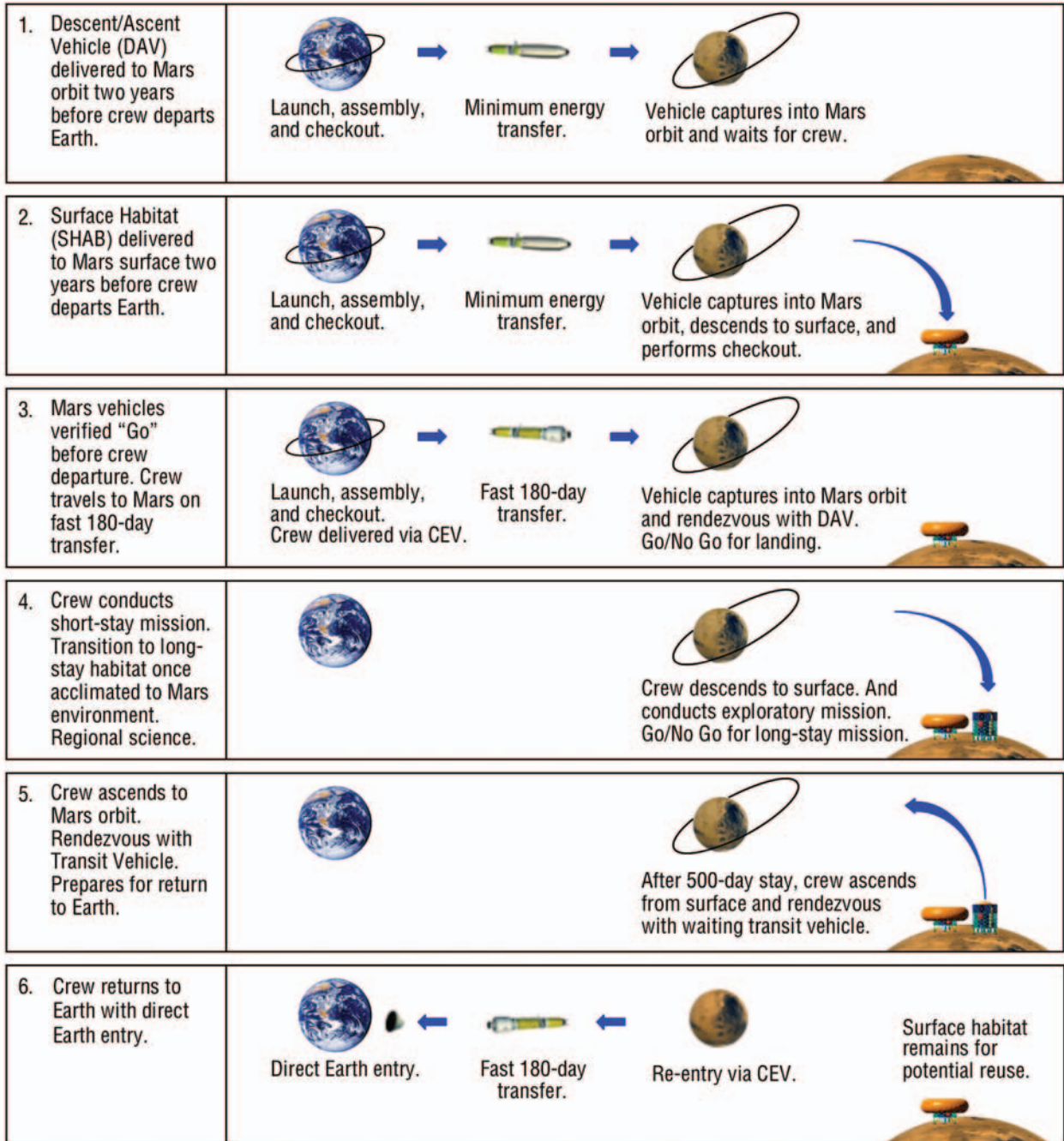
Figure 2-8. Mars Exploration DRM
