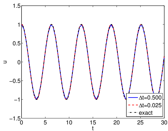
(d) Four-stage Runge-Kutta
