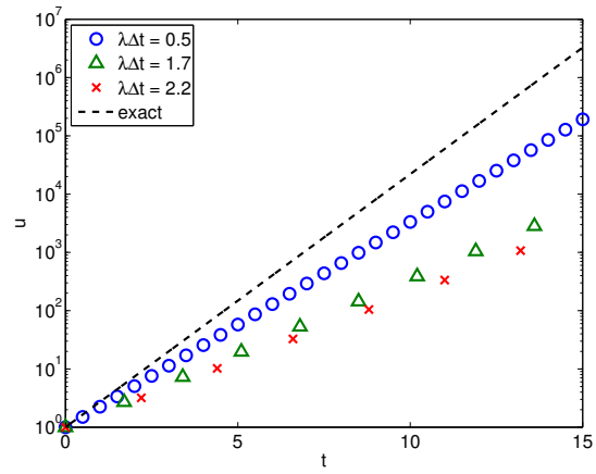
(d) solution ( \lambda = 1 )
