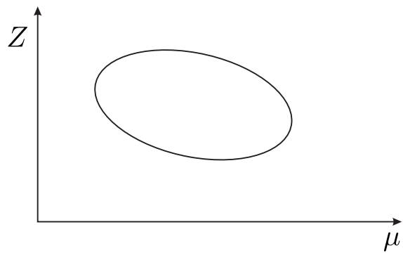
(d) isola
