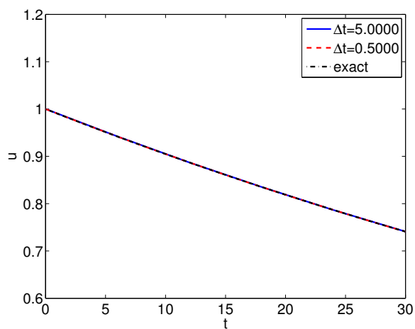
(d) Crank-Nicolson
